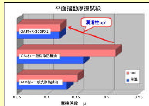
平面摺動摩擦試験機による プレトンR-303PX2潤滑性評価試験データ
