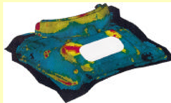
板材の成形シミュレーション (クォーターインナパネル板厚減少率解析結果)
